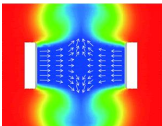
気流シミュレーション図
